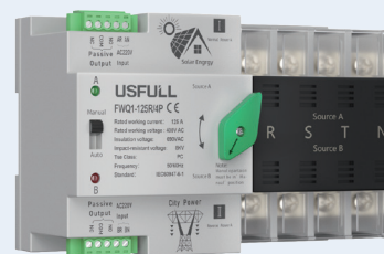
ATS
