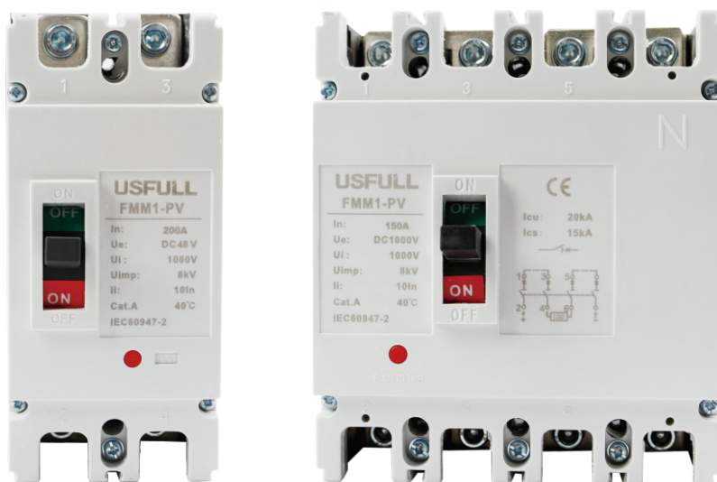
FMM1-PV DC Breaker (DC MCCB)
